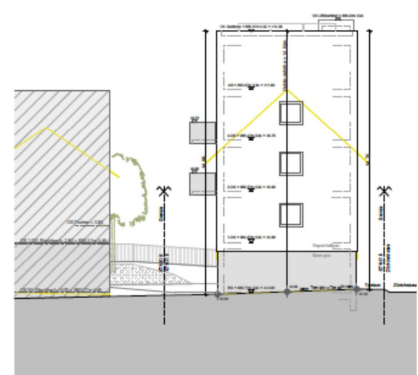
Ansicht Nord
